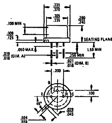
TO-5
